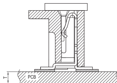
PCB ASS'Y
